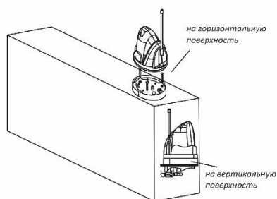
Рис. 1 Варианты монтажа
