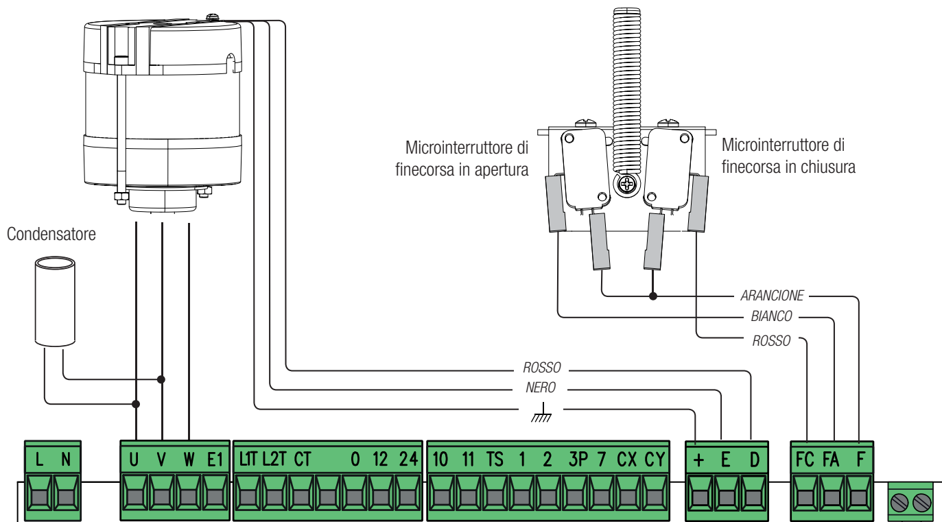
Finecorsa meccanico
