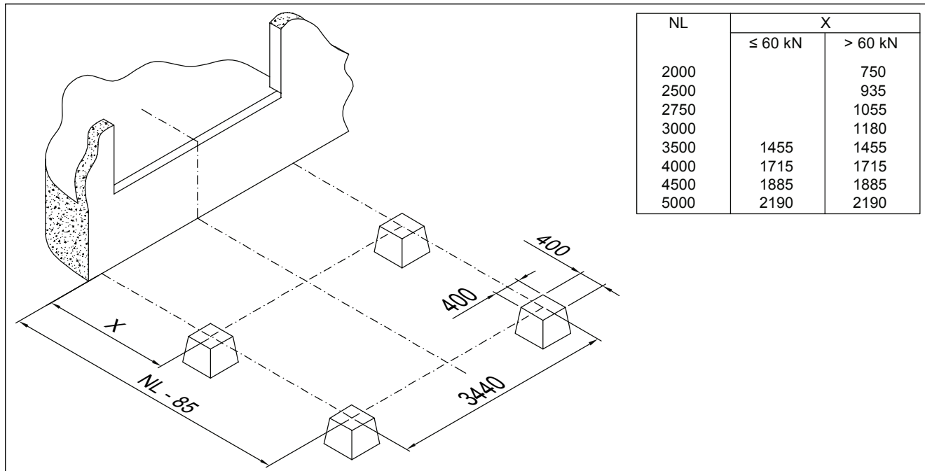
Рис. 4: Фундамент PS2
