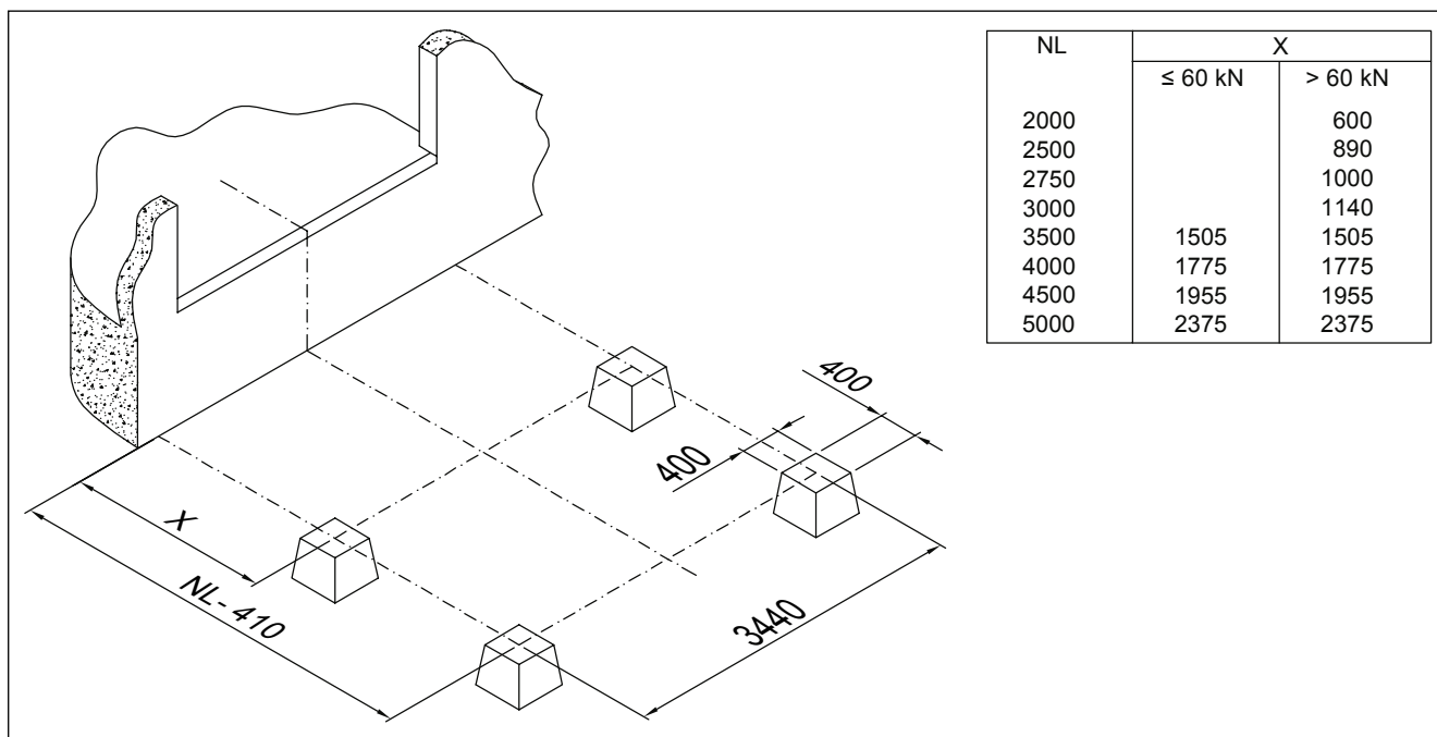
Рис. 5: Фундамент PT2
