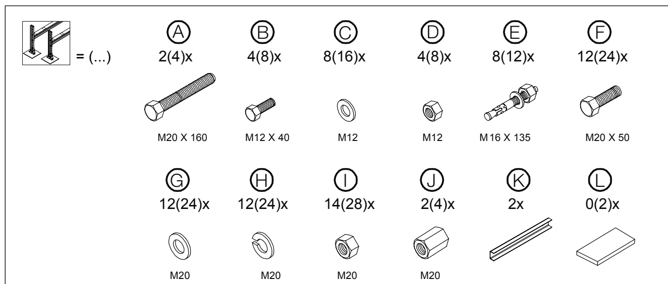
Рис. 2: Комплект поставки / монтажный материал
