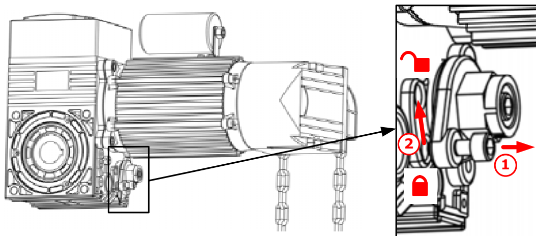
Рис. 4. Ручная разблокировка
